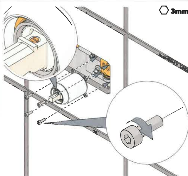
Skruva i insatsen med en 3 mm insexnyckel.
