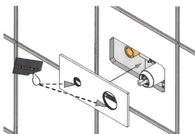
Fetta in o-ringarna i täckplattans hål med bifogat fett.
