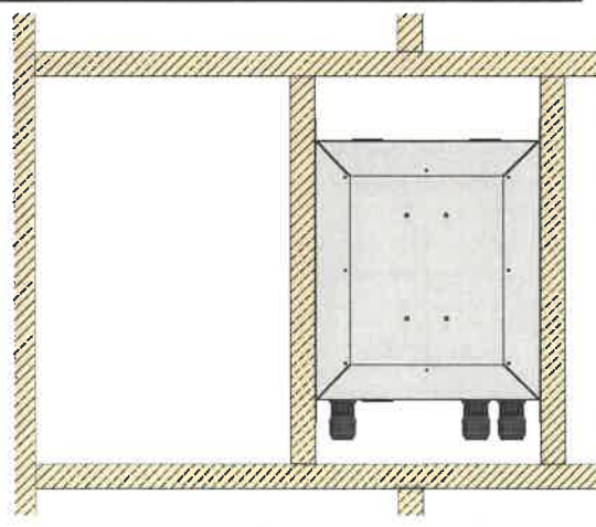
Exempel på väggmontage
